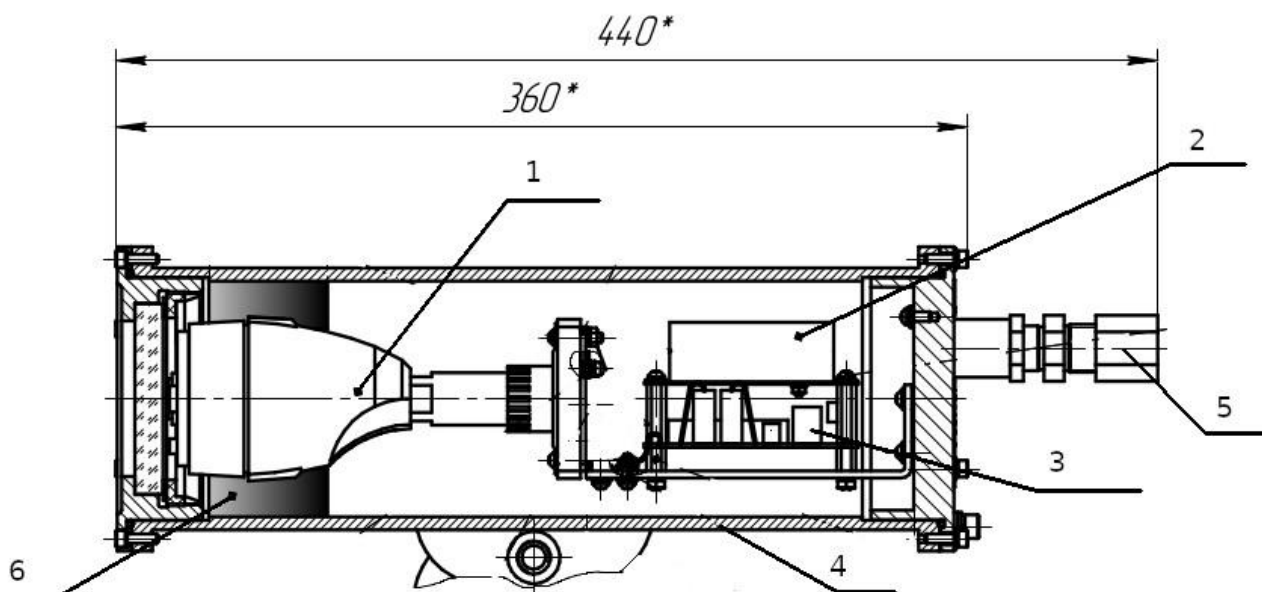
Рис. 2 Конструкция БВК-РВ ВEW-1ТХ-АARFRZ-35.75
