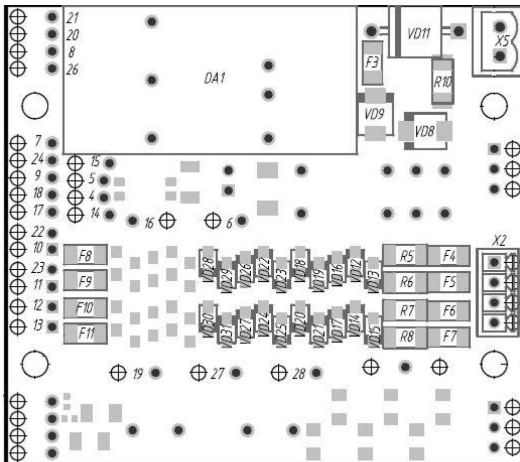
Рис. 3 Модуль искрозащиты
