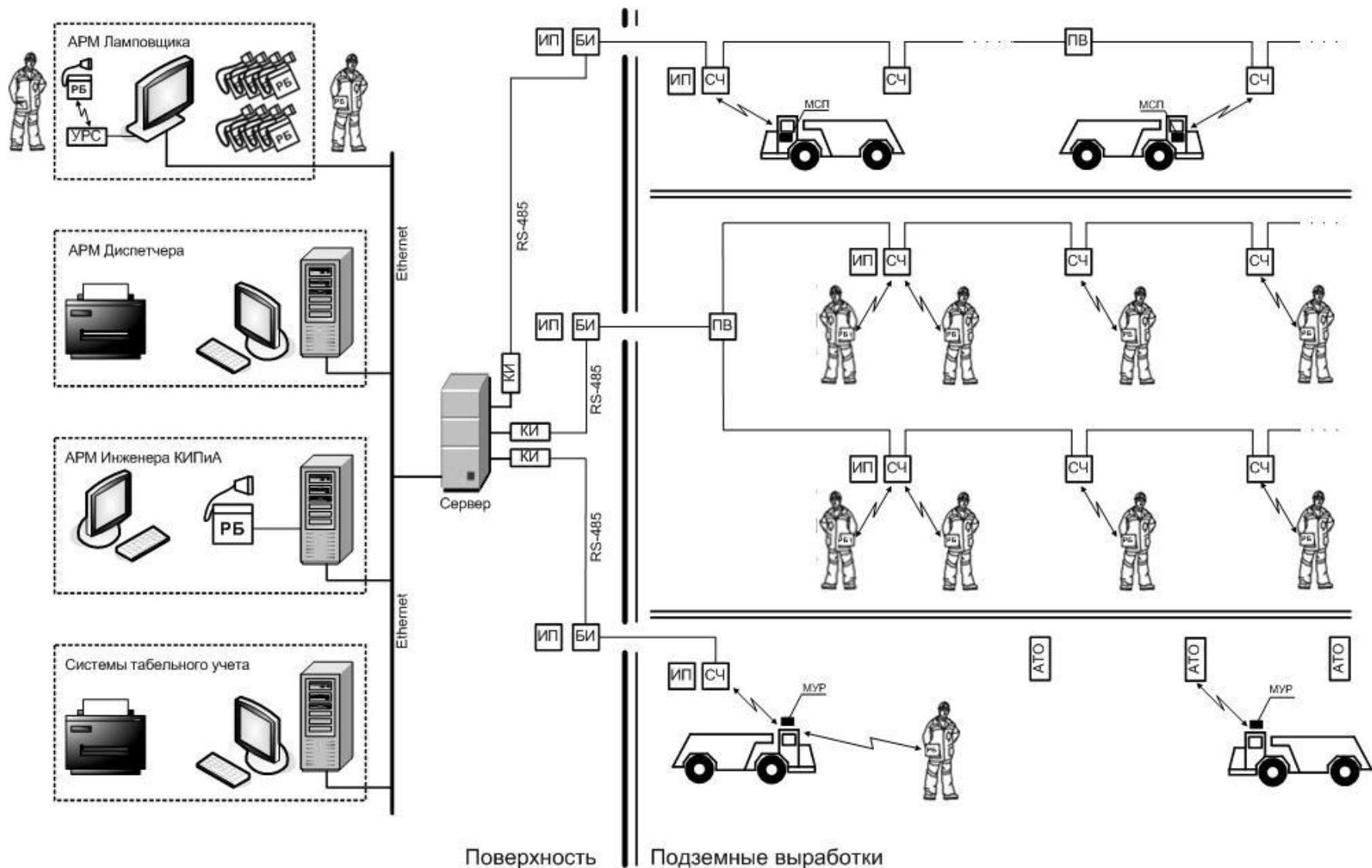
Рисунок 1 – Структура Системы СПГТ-41:
