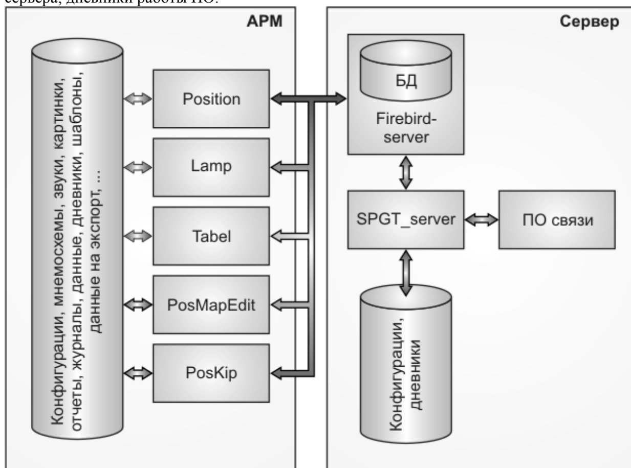
Рисунок 2 – Структура программного обеспечения
